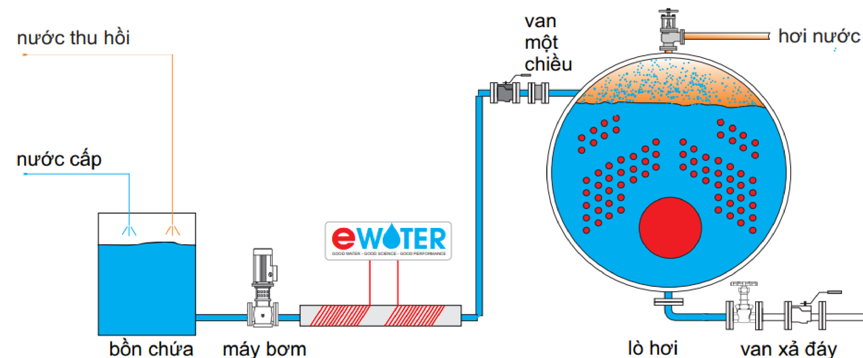
Sơ đồ lắp đặt thiết bị xử lý cặn cho lò hơi
